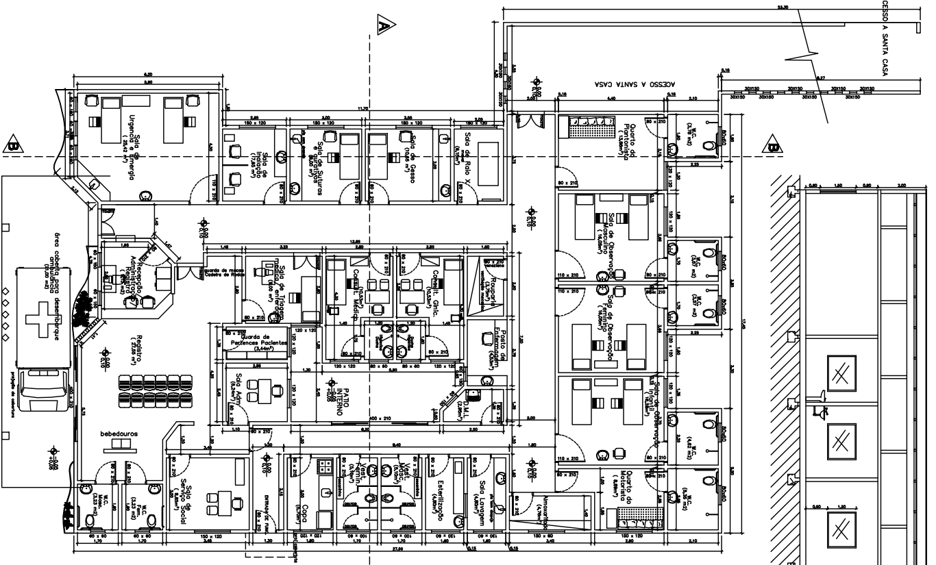
PLANTA BANDA ESC 1/50
