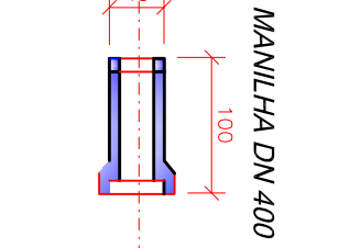
DET. LONGIT.
